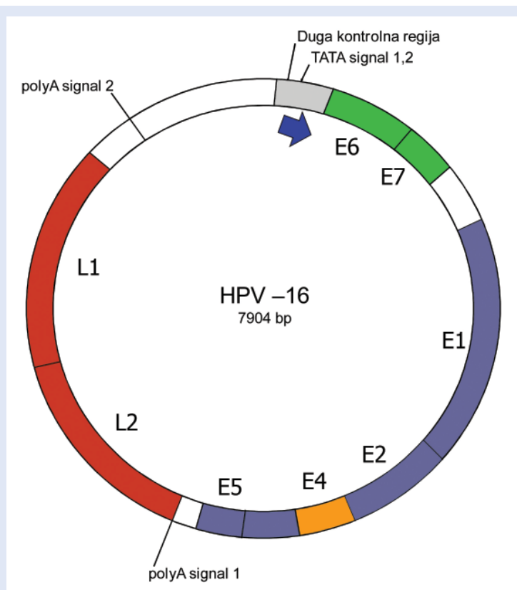
Slika 2. Organizacija genoma humanog papiloma virusa (HPV); genom HPV-a je kružna dvolančana DNA, dužine oko 8.000 parova baza; genska mapa sadrži 6 ranih ( Early ) gena, E1 do E7 – regulatorni geni izraženi u različitim fazama diferencijacije epitelnih stanica, 2 kasna ( Late ) gena, L1 i L2 – strukturni geni, koji su izraženi u stanicama gornjeg epitela, u kojima se replicira virusna DNA i LCR ( Long Controlling Region ) – duga kontrolna regija
