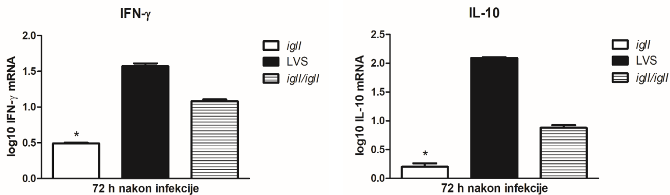
Slika 10. Razina mRNA citokina IFN- \gamma i IL-10 u plućima miševa 72 sata nakon infekcije s F. tularensis soj LVS, mutantom \Delta igII i njenom komplementatom igII/igII. *Rezultati prikazuju statistički značajnu razliku u sintezi citokina IFN- \gamma i IL-10 u tkivu pluća miševa inficiranih mutantom igII i F. tularensis subsp. holarctica LVS. Razina od p < 0,05 smatrana je statistički značajnom
