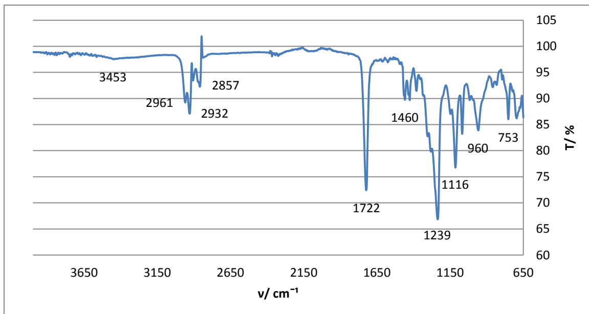
Slika 20: IR spektar uzorka 1 termički starenog 1 dan pri 90 ° C.
