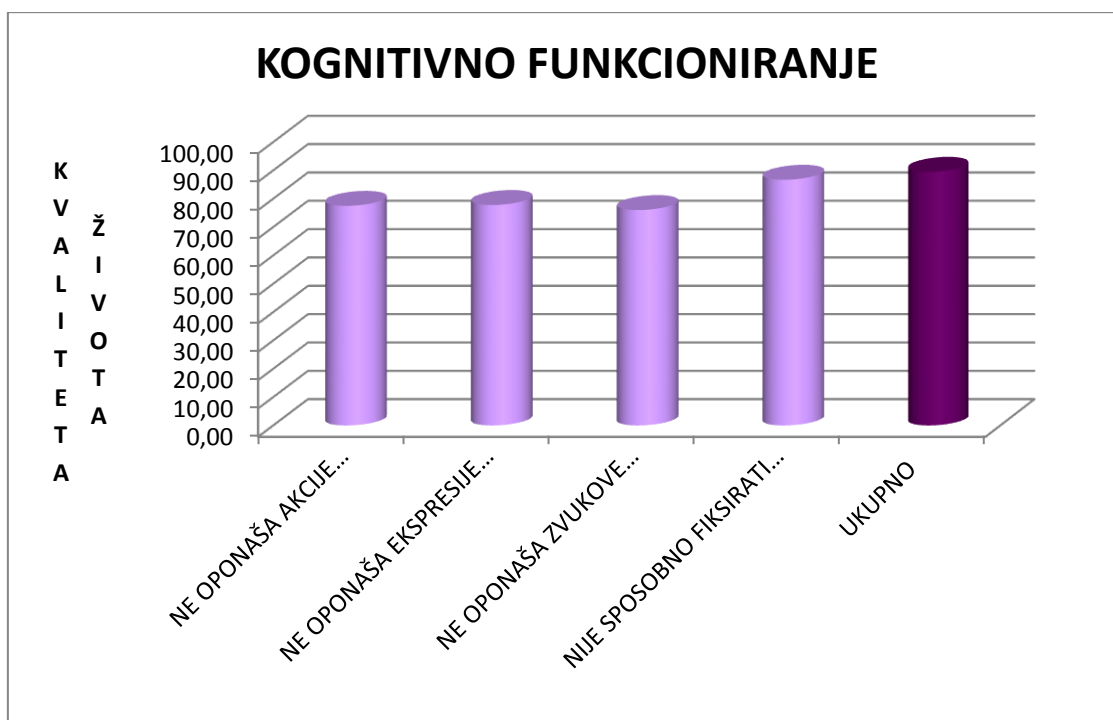
Slika 7. Kognitivno funkcioniranje
