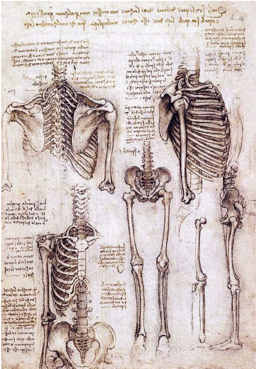
Slika 4: Koštani sustav
