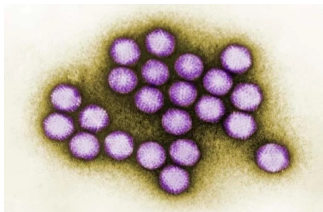
Slika 7. Adenovirus
