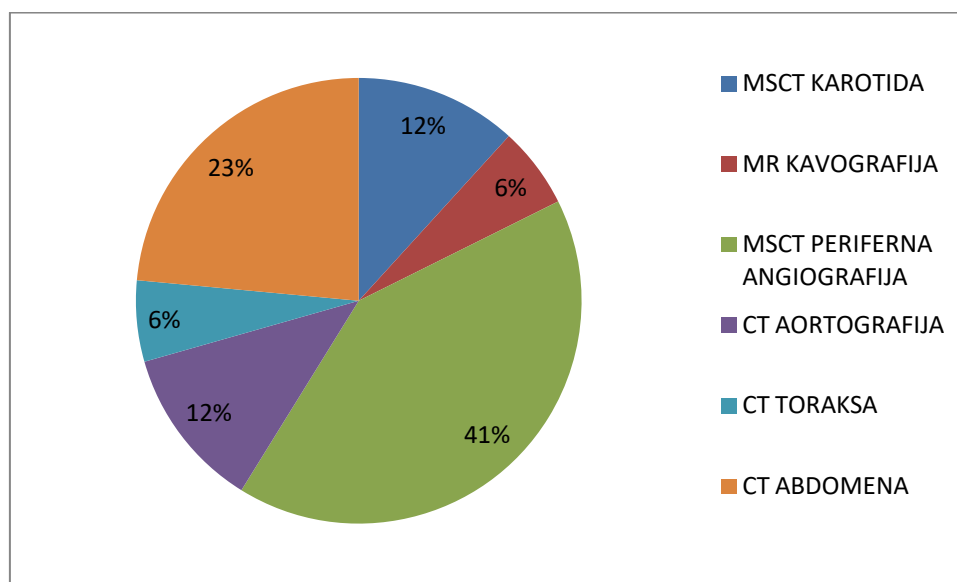
Slika 1. Kontrastne pretrage
