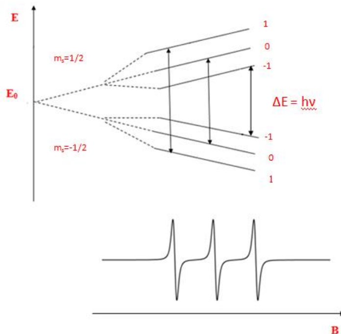
Slika 6. Energijske razine nitroksilnog radikala u magnetskom polju.
