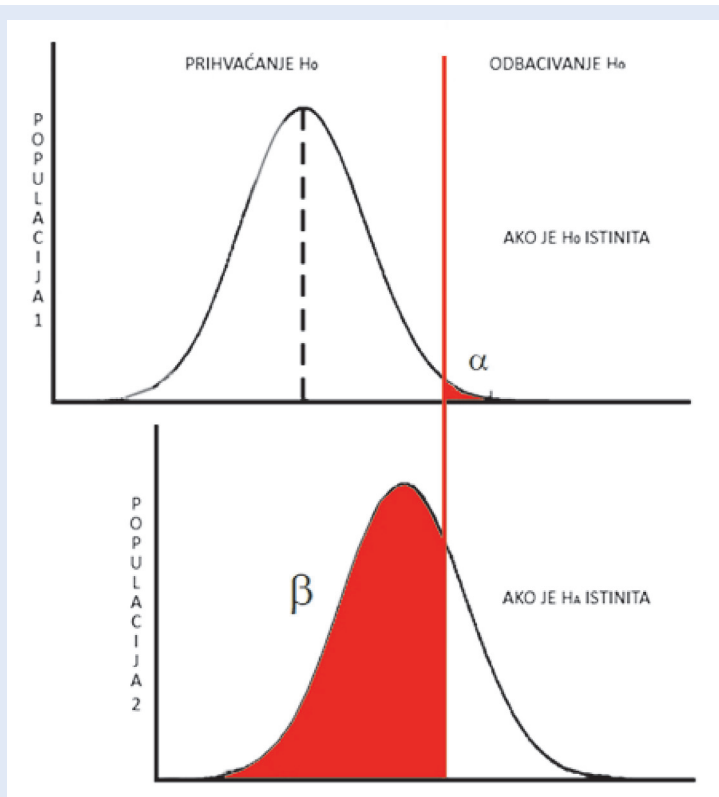
Slika 2. Ilustracija slučajne pogreške tipa I i II. Pretpostavimo da postoje dvije populacije s različitim srednjom vrijednošću mjerene varijable, ali čije se normalne krivulje raspodjele međusobno djelomično preklapaju. Ako je nul-hipoteza ( H_0 ) istinita, odnosno nema značajne razlike između uspoređivanih populacija, tada postoji mala vjerojatnost da će stvarna srednja vrijednost ispitivane varijable biti desno od vertikalne linije, odnosno u zacrnjenom području (pogreška tipa I ili \alpha ), tj. postoji mala vjerojatnost pogrešnog odbacivanja istinite H_0 . Ako je alternativna hipoteza ( H_a ) istinita, tada postoji više od 50 % vjerojatnosti da će srednja vrijednost biti lijevo od vertikalne linije i H_0 neće biti odbačena, iako bi trebala, što predstavlja pogrešku tipa II ili \beta . Ako je \beta = 0,67 , tada je vjerojatnost da ćemo točno utvrditi postojanje stvarne razlike između mjerene varijable dviju populacija 1 - \beta = 0,33 , odnosno 33 % (prilagođeno prema ref. 12).
