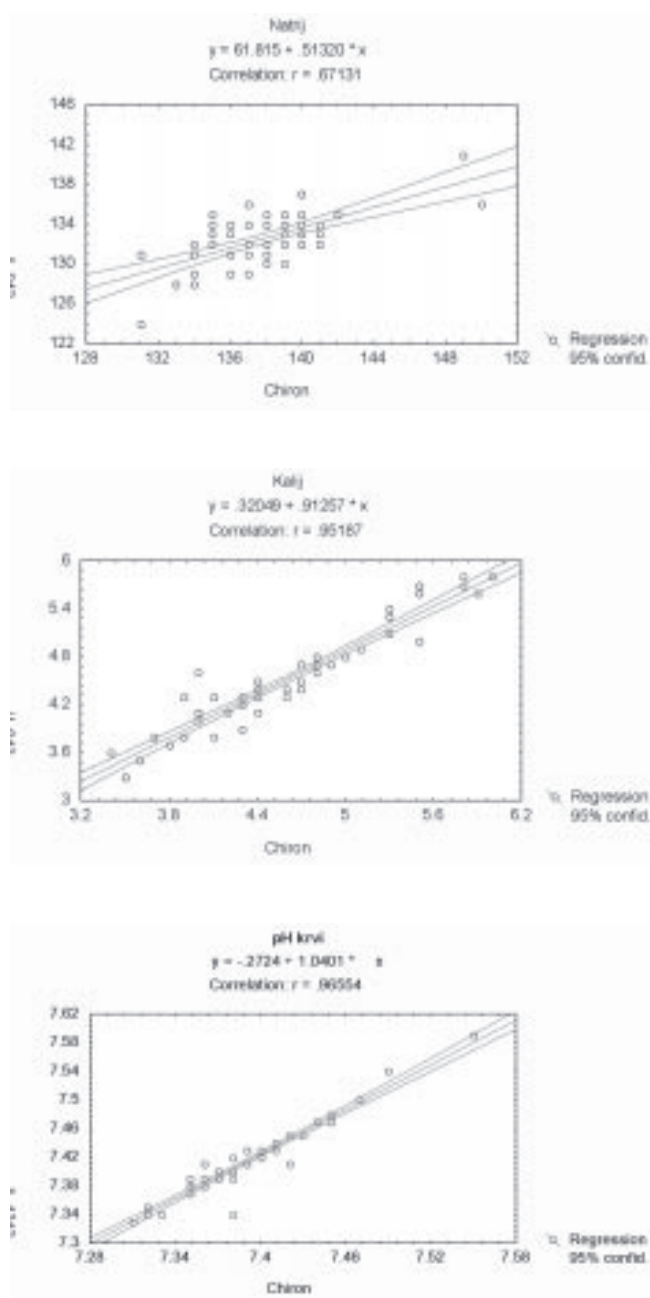
Slika 1. Korelacije u mjerenju koncentracije natrija, kalija (mmol/L) i pH aparatom Chiron i IL-943, odnosno 1312.
