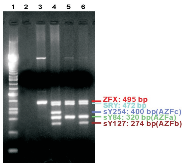
Slika 2. Prikaz multipleks-A reakcije u kontrolnih ispitanika i dvojice ispitanika s mikrodelecijama kromosoma Y
