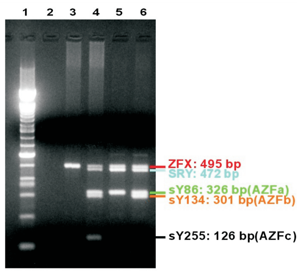
Slika 3. Prikaz multipleks-B reakcije u kontrolnih ispitanika i dvojice ispitanika s mikrodelecijama kromosoma Y
