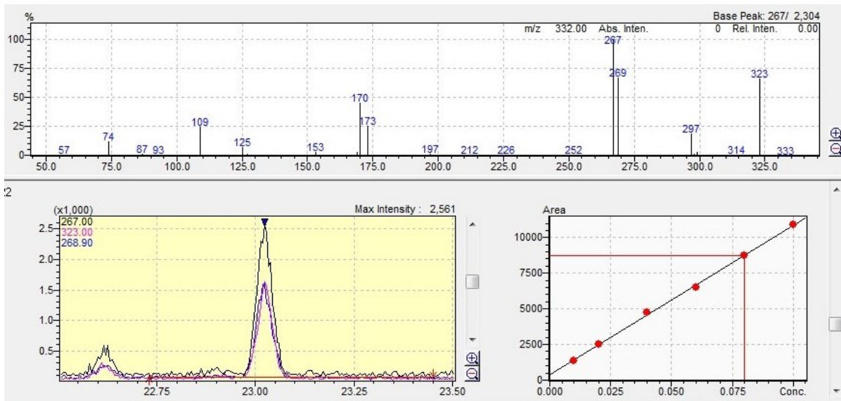
Slika 17. Klorfenvinfos GC – MS
