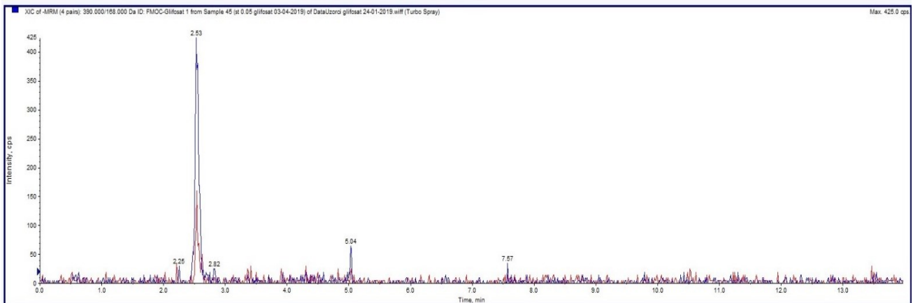
Slika 20. Izgled kromatograma standarda glifosata na LC – MS/MS
