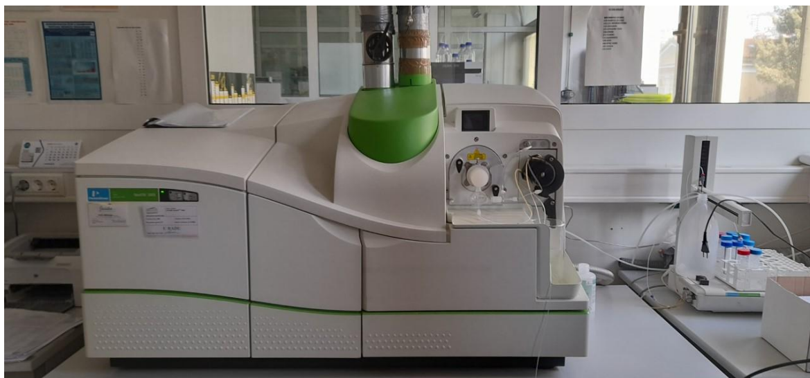
Slika 7. ICP - MS NexION 300x Perkin Elmer
