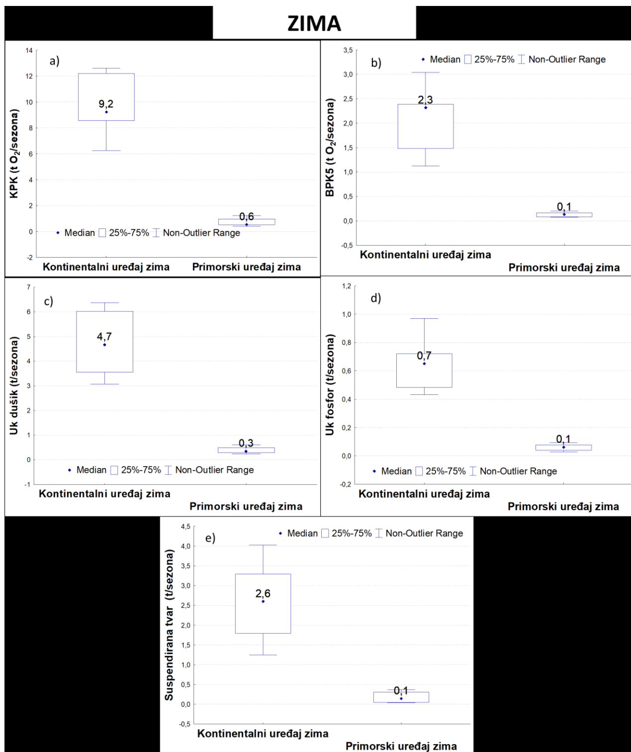
Slika 43. Rezultati Mann-Whitney U testa zimskog opterećenja recipijenta kontinentalnog i primorskog uređaja za a) KPK b) BPK 5 c) ukupni dušik (Uk N) d) ukupni fosfor (Uk P) e) suspendiranu tvar (Susp. tvar)
