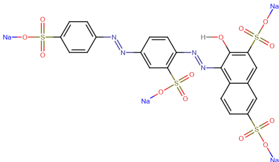
Slika 11. Kemijska struktura azo boje Ponceau S.
