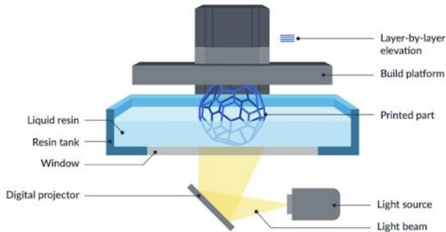
Slika 3. Prikaz principa rada i dijelova 3D pisača temeljenog na VP tehnologiji (22). (Preuzeto iz: Nexa3D.com. What is mSLA? The Ultimate mSLA 3D Printing Guide; Dostupno na: https://nexa3d.com/blog/msla-3d-printing )
