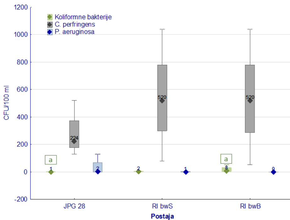
Slika 14. Usporedba koncentracija koliformnih bakterija, C. perfringens i P. aeruginosa u vodenom stupcu ovisno o postaji s prikazom medijana ( \diamond ), 25 % - 75 % percentila ( \square ) i raspona rezultata bez ekstrema ( \top ). Lokacije označene istim slovima statistički se značajno razlikuju ( p < 0,05 ).
