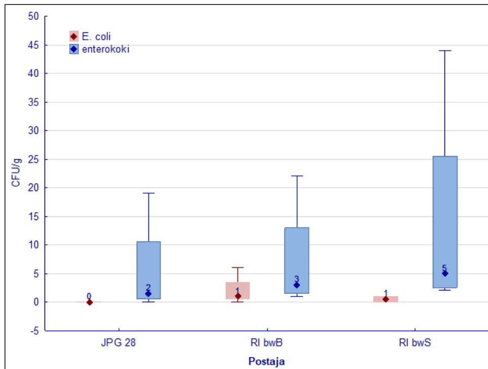
Slika 7. Razina E. coli i crijevnih enterokoka analiziranih u uzorku sedimenta ovisno o mjestu uzorkovanja s prikazom medijana (◇), 25 % - 75 % percentila (□) i raspona rezultata bez ekstrema (⌈). Lokacije se statistički značajno ne razlikuju ( p > 0,05 ).
