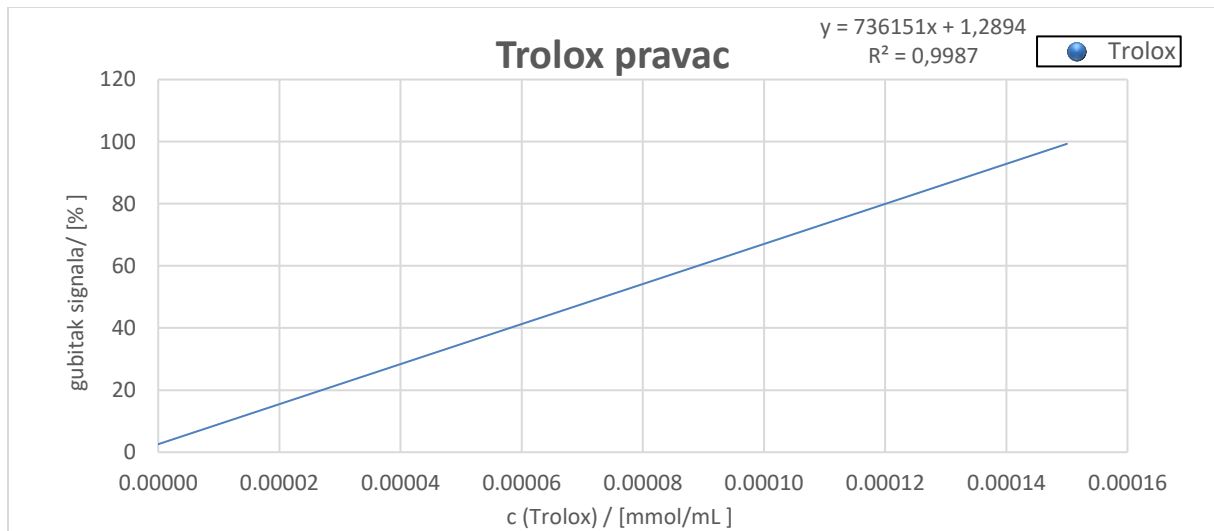
Slika 9. Baždarni pravac Trolox-a
