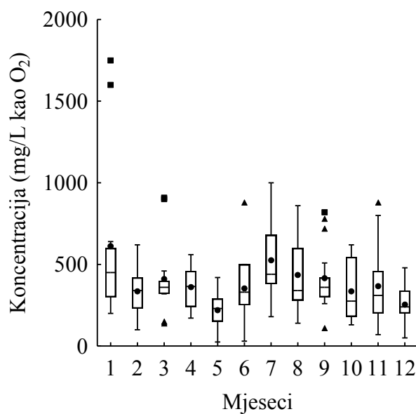
Slika 6. Koncentracije BPK5 u otpadnoj vodi tijekom pet godina ispitivanja grupirane po mjesecima. Prikazan je box-wisker graf koji sadrži 25ti i 75ti percentil (box □), raspon podataka bez ekstremata i outliera (wisker T ⊥ □), medijan (—), srednja vrijednost (●), outlier (▲) i ekstrem (■)
