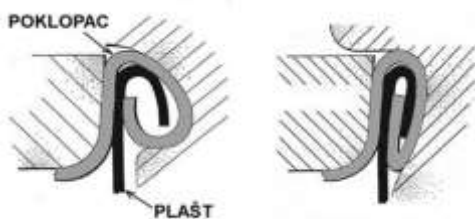
Slika 6.6. Hermetičko zatvaranje limenki strojnim oblikovanjem dvostrukog šava (preuređeno prema 8 )
