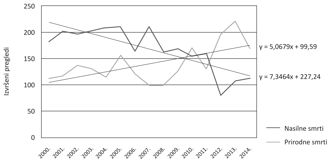
Slika 1. Grafički prikaz razlike u učestalosti prirodnih u odnosu prema nasilnim smrtima. Prikazani su i pravci koji predstavljaju linearni trend za obje varijable. Negativan trend može se opaziti za nasilne smrti, dok je trend pozitivan za prirodne smrti.
