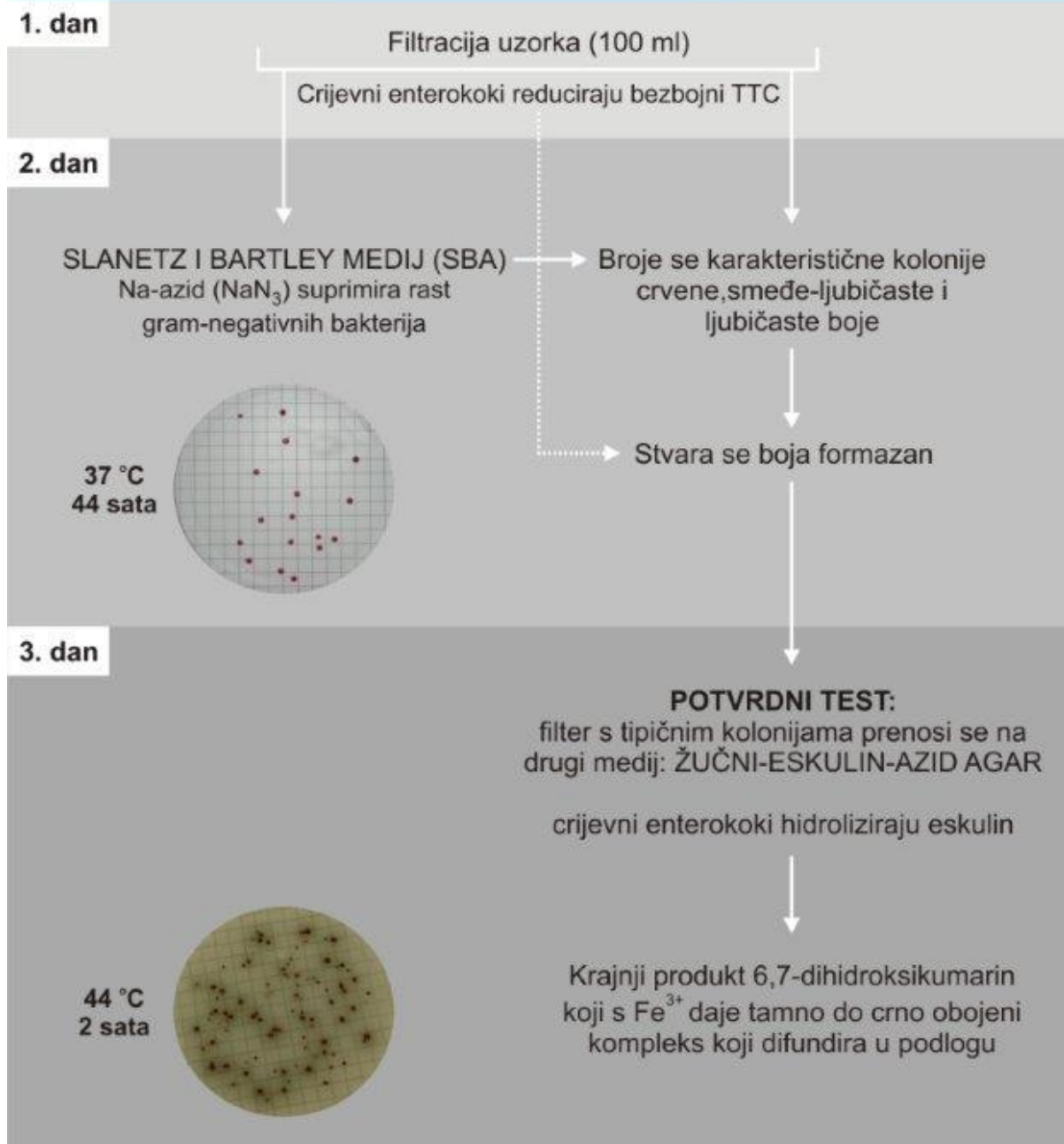
Slika 6. Metoda membranske filtracije fekalnih streptokoka (HRN EN ISO 7899-2:2000)
