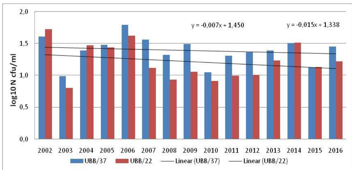
Slika 8. Trend kretanja broja kolonija pri temperaturama od 22°C i 37°C tijekom razdoblja 2002. – 2016.
