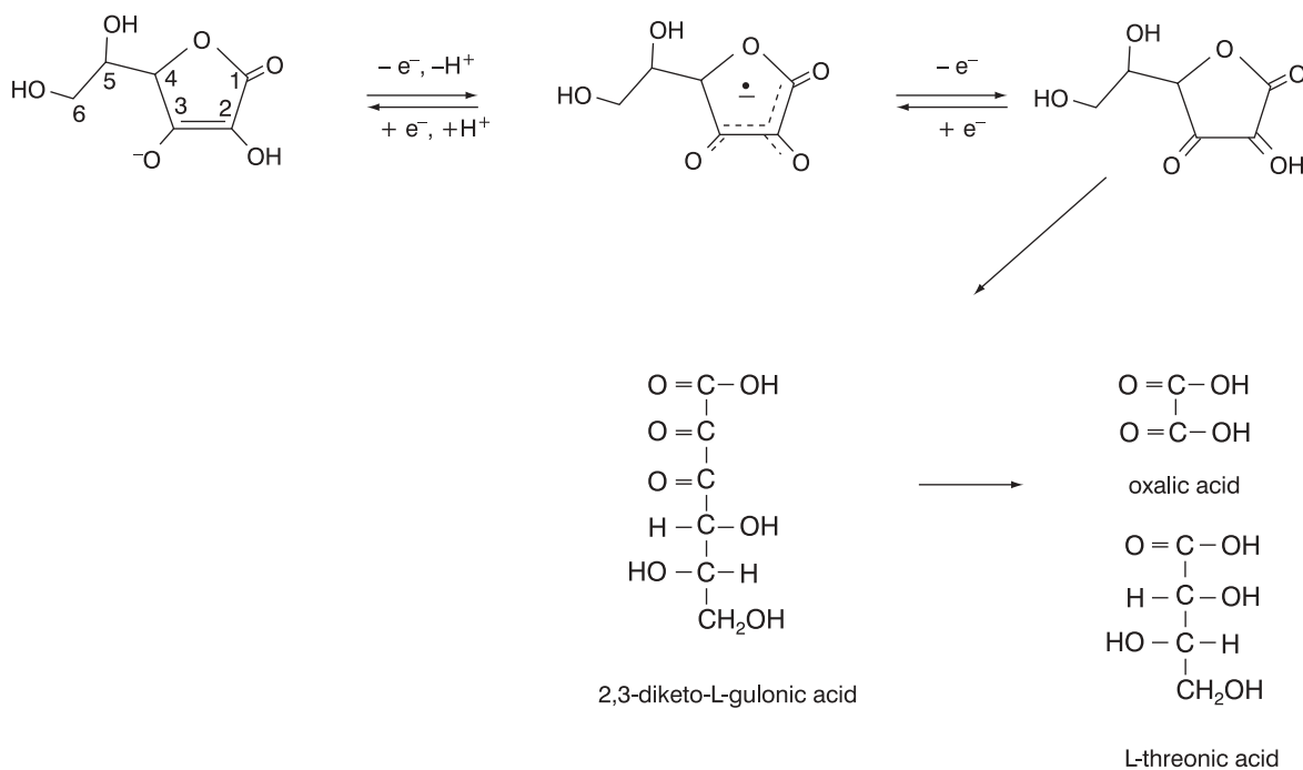
SLIKA 3. Razgradnja askorbata.
